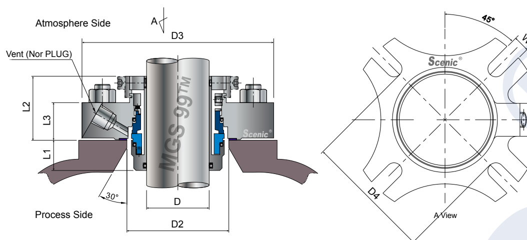
MGS® 99™ - 公制標準尺寸
